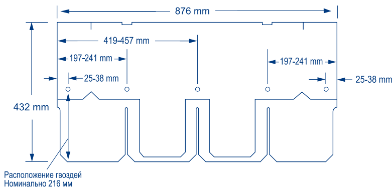
Стандартная схема крепления - пять гвоздей на черепицу
