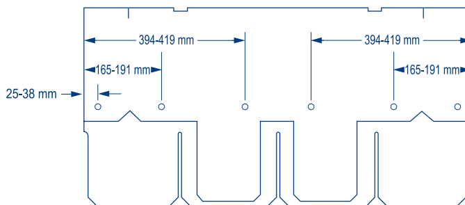
Схема крепления шестью гвоздями – где требуют местные нормы
