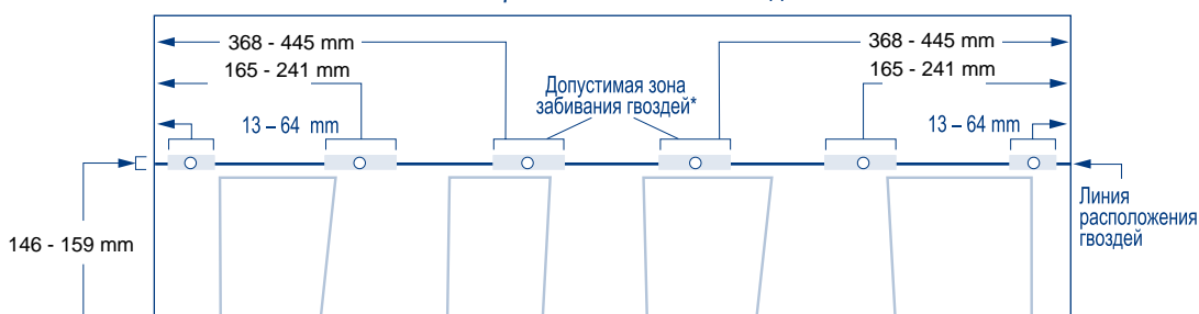
Схема крепления шестью гвоздями
